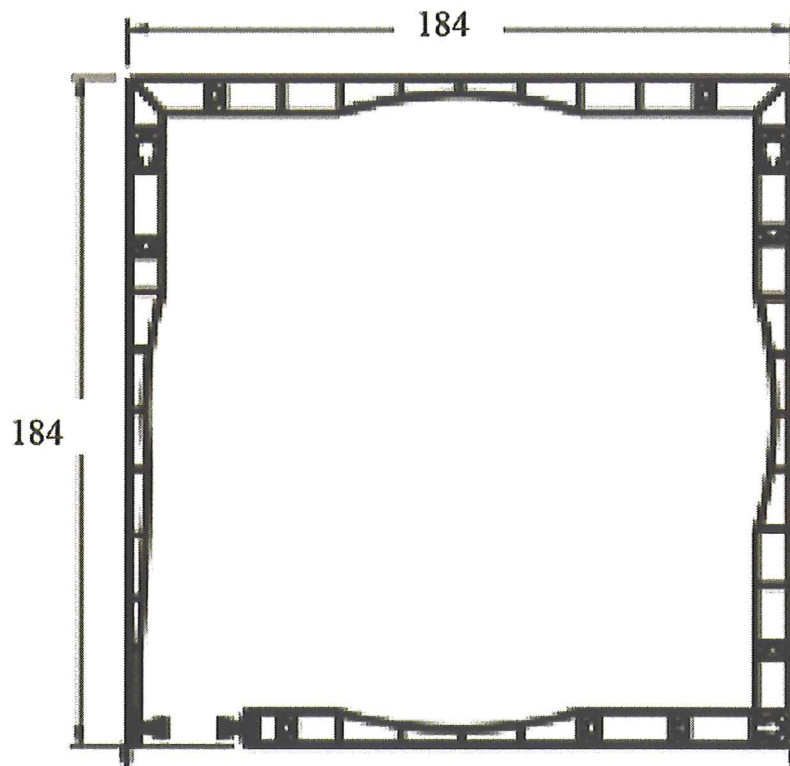
SECCION DEL CAJON DE PVC “DOBLE TABIQUE”
